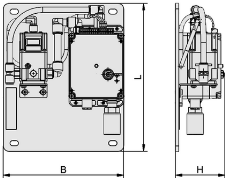
设计参数 SRCU-Mini-P-M
