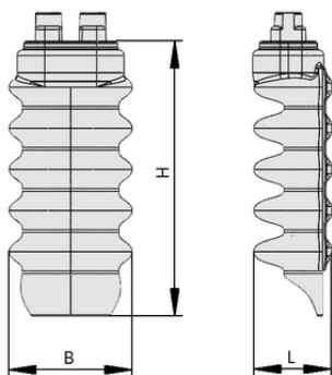
设计参数 FINGER-SPARE-UNIT 6C
