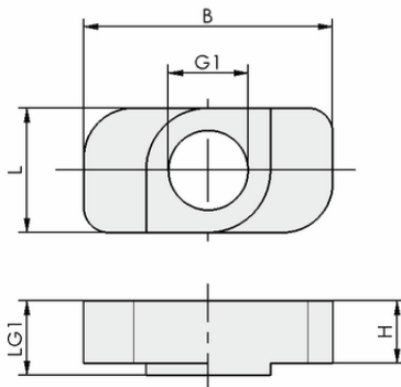
设计参数 NUT-STEI 10x20 M8-IG
