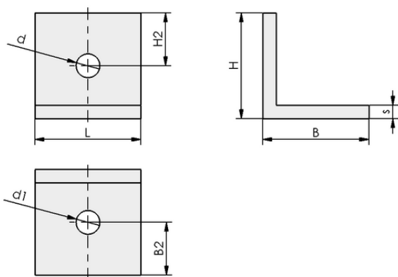
设计参数 BEF-WIN 40x40x40 5 MO-PROF
