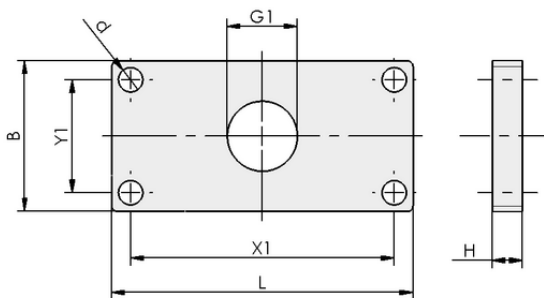
设计参数 VRS-PL-80x40 G1/2-IG MO-PROF
