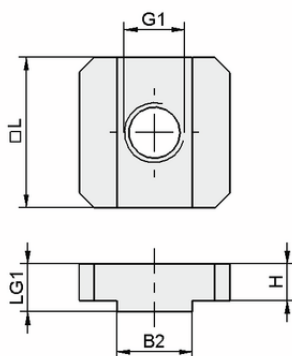
设计参数 NUT-STEI 20x20 M6-IG 10
