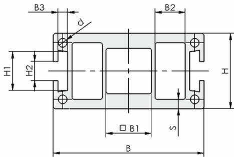
设计参数 MO-PROF 80x40 2TN AL-1
