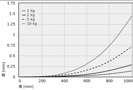
变形管 60 x 5 毫米
